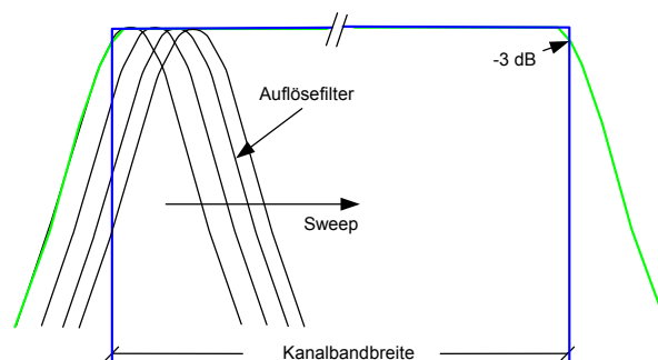
Bild 2.18 Approximation des Kanalfilters durch Sweepen mit kleiner Auflösungsbandbreite
