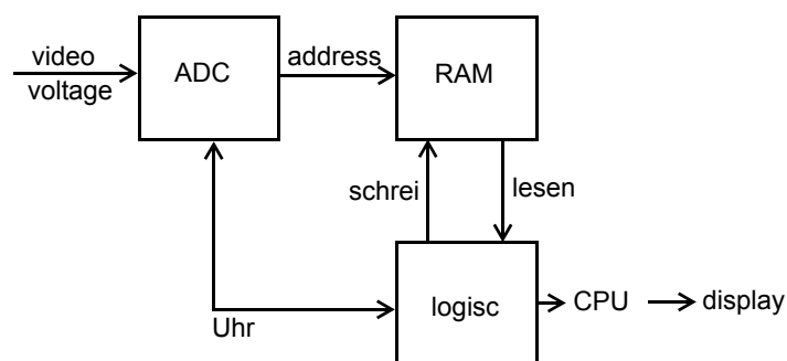
Bild 4.11 Prinzipschaltbild zur Messung der Amplituden-Wahrscheinlichkeitsverteilung (APD)
